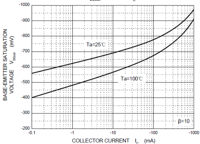
V_{BEsat} — I_C
