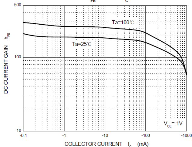
h_{FE} — I_C
